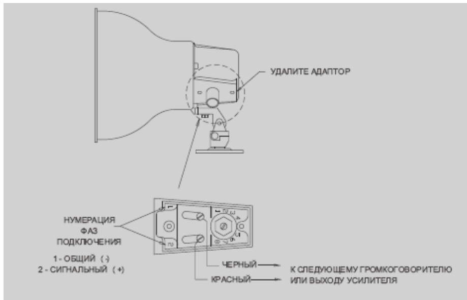
Схема 3: Подключение
