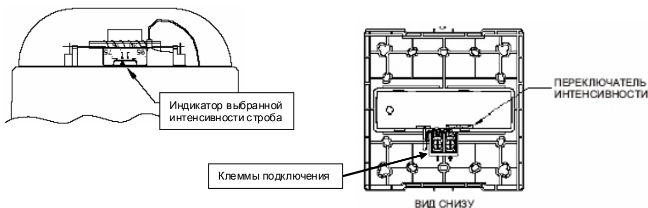
Рис 2: Расположение переключателя выбора интенсивности строб-вспышки.
