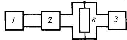
1 — испытуемый ТА; 2 — питающий комплект; 3 — осциллограф; R — резистор с сопротивлением (600 \pm 60) Ом, мощностью не менее 0,25 Вт
