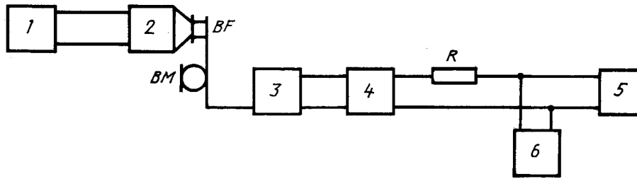
1, 6 — электронные вольтметры переменного напряжения; 2 — ухо искусственное; 3 — испытуемый телефонный аппарат; 4 — питающий комплект; 5 — генератор сигналов низкочастотный; BF — телефон испытуемого ТА; BM — микрофон испытуемого ТА; R — резистор сопротивлением (600 \pm 60) Ом, мощностью не менее 0,25 Вт
