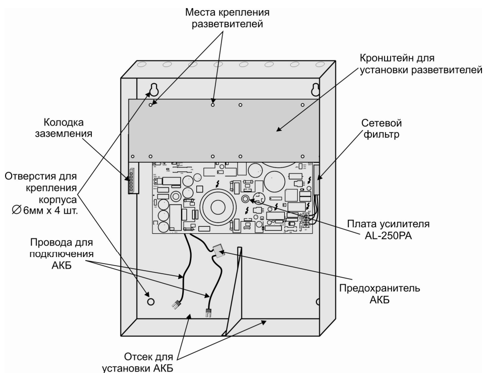
Рис 2. Общий вид усилителя AL-250PA (без передней двери)
