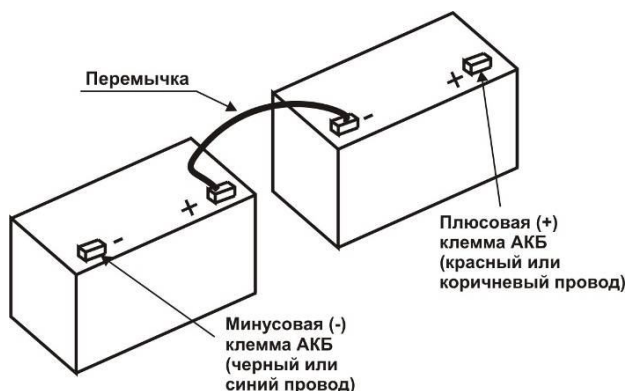
Рис.10 Размещение батарей и их подключение
